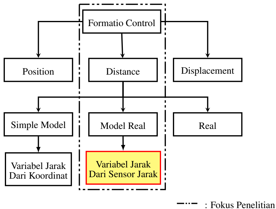
Gambar 3.1: Kerangka Penelitian
